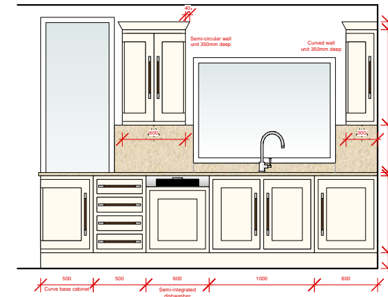
ELEVATION B
